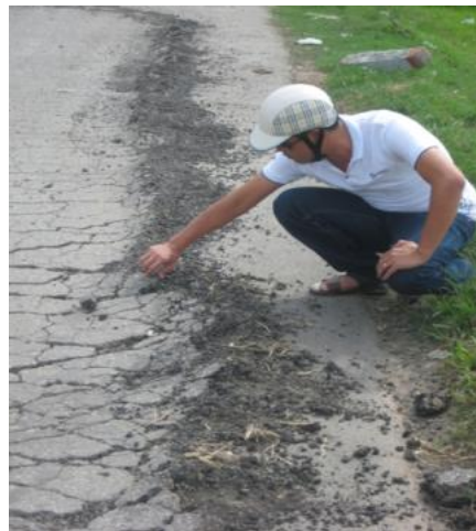
Chỉ cần lấy tay là có thể bóc được cả mảng lớn nhựa đường
